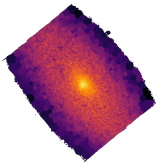
IC3392
