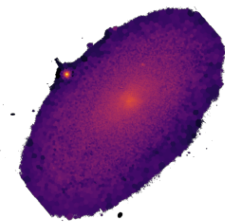
NGC4298
