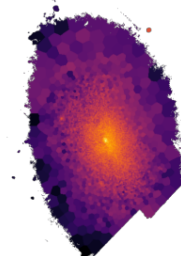
NGC4501
