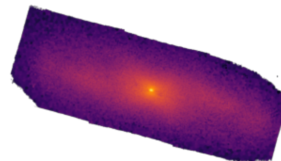
NGC4293
