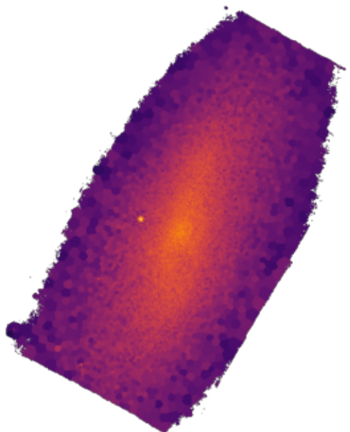
NGC4064
