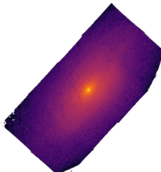
NGC4501
