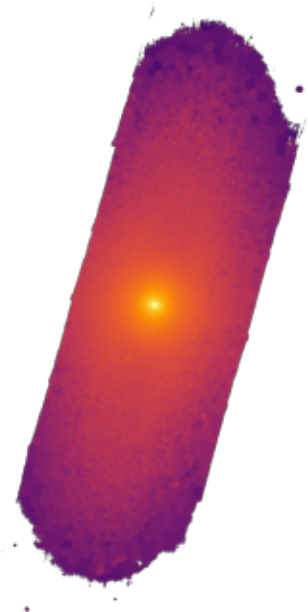
NGC4698
